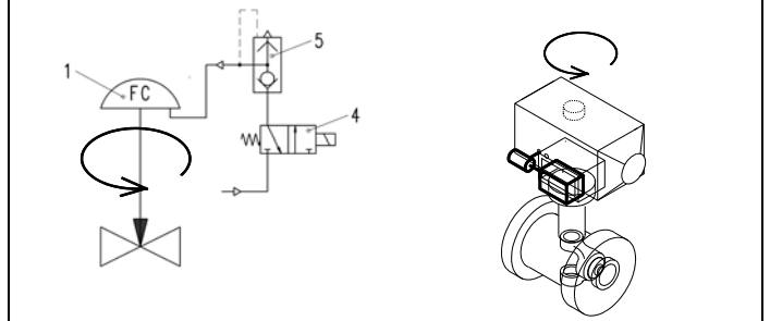
Bild 5 - Wirkbild bei Ausführung mit Magnetventil und Schnellentlüftung – die Sicherheitsstellung ist – Ventil zu – Die Feder hält die Armatur geschlossen
